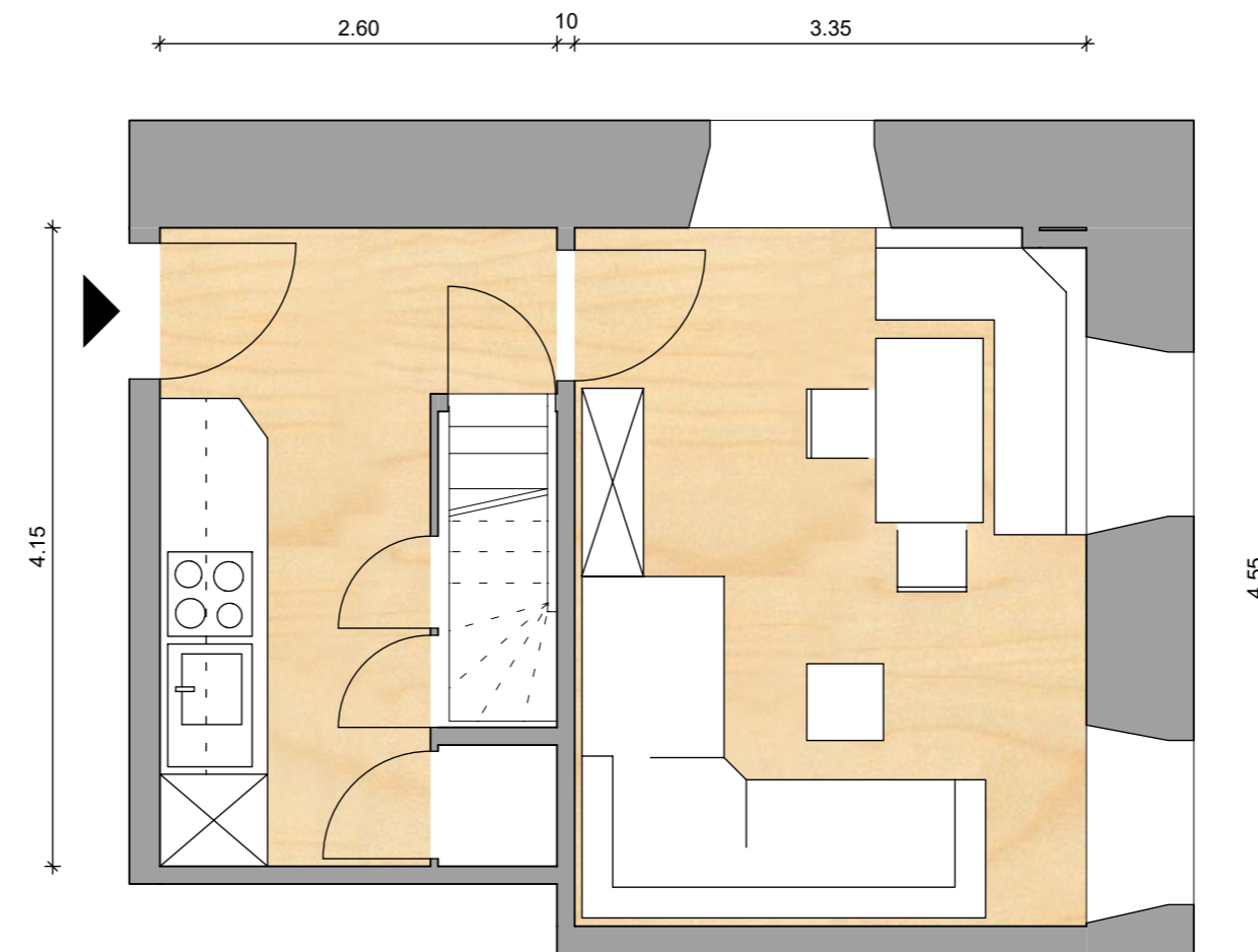
Grundriss Erdgeschoss 1:50
