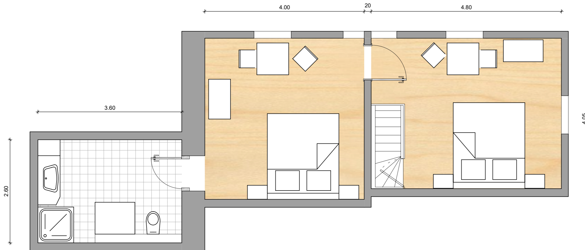
Grundriss Obergeschoss 1:50
